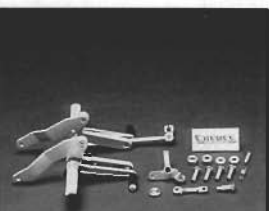
●コースフィクスドレーシングステップ 55ミリバック+50ミリアップ 32,000円
